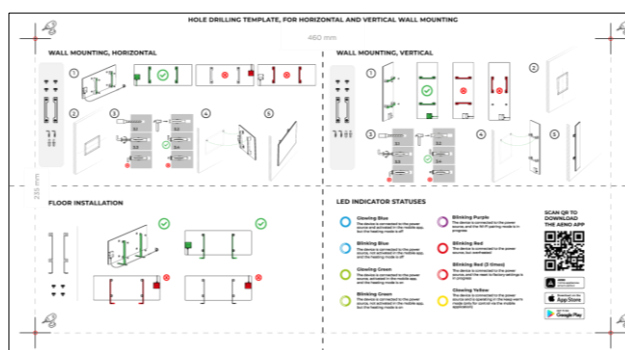
5 – Sjabloon voor het boren van gaten in de muur
