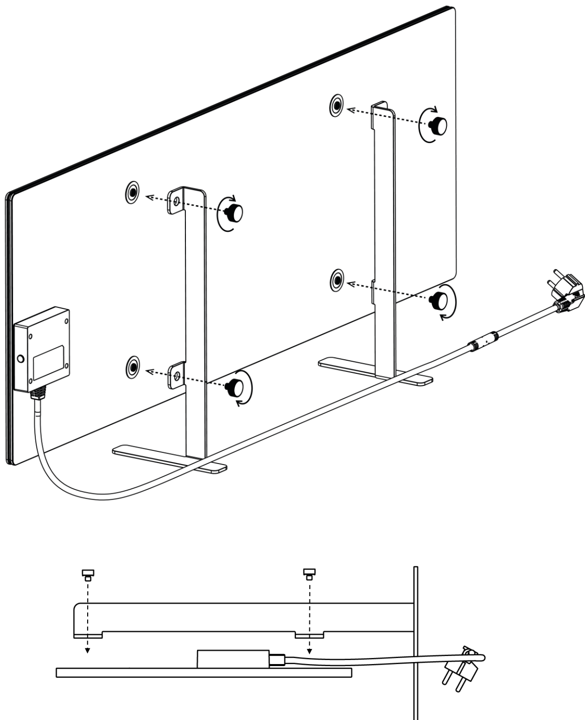
Figuur 7 – Voetbevestiging (op de vloer)
