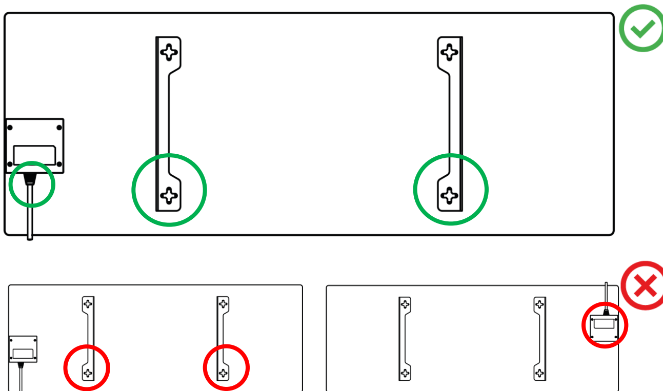
Figuur 8 – Installeren van de beugels
